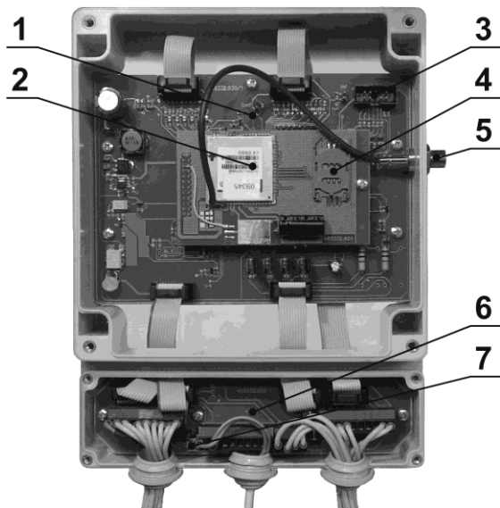
Рис. 1. Контроллер Индел 1708.1 со снятыми панелями.
