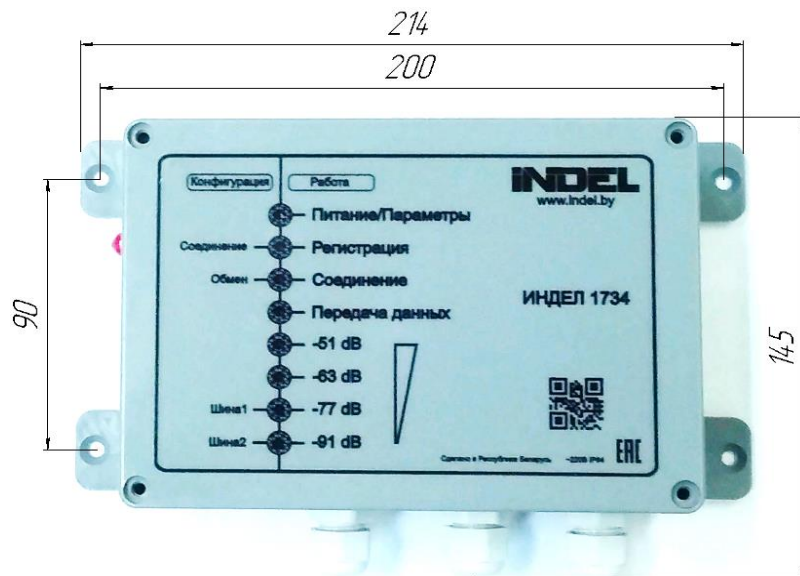
Рис.2 Габаритные и присоединительные размеры устройства
